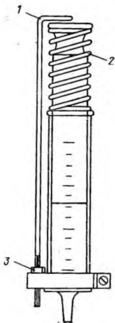
Рис. 8.2. Дозатор.
