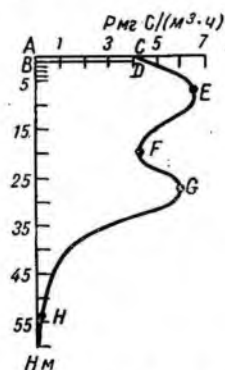
Рис. 8.5. Пример кривой самопоглощения 14 BaCO 3 ( R = 9000 имп/мин).
