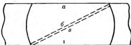
Рис. 5.2. Раскрой сетки. Сшиваются детали a с b , b с g [10].
