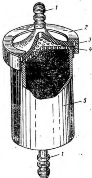
Рис. 7.1. Фильтр Зейтца для фильтрации проб на хлорофилл.
