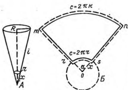
Рис. 5.1. Выкройка сетяного конуса для планктонной сетки [10].
